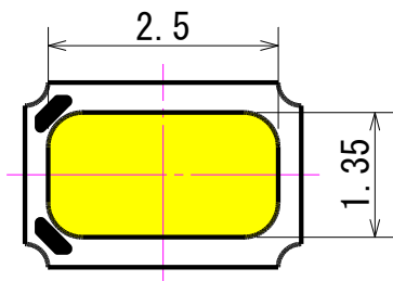
図3. LEDの発光面サイズ
