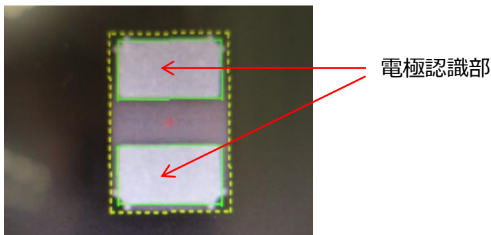
図8. 電極端子認識 (推奨)
