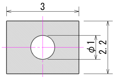
図2. 吸着ノズル先端部形状
